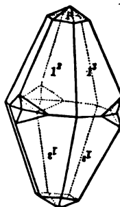
Calcite.
